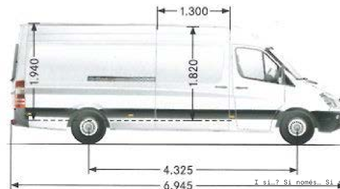
SECCIÓ LONGITUDINAL DRETA
