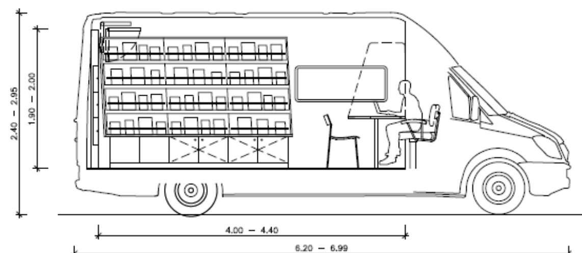
SECCIÓ LONGITUDINAL ESQUERRA
