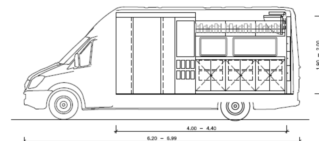
SECCIÓ LONGITUDINAL DRETA
