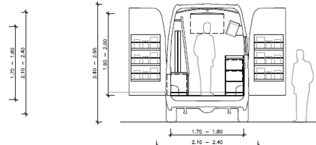
SECCIÓ TRANSVERSAL
